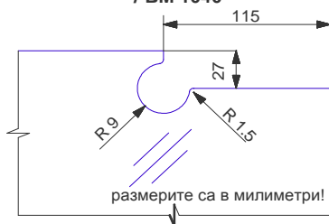
ИЗРЕЗИ НА СЪКЛОТО ЗА ВМ 1010 / ВМ 1020 / ВМ 1030 / ВМ 1040
