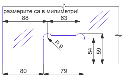
ИЗРЕЗИ НА СЪКЛОТО ЗА ВМ 1099
