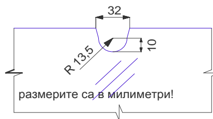
ИЗРЕЗИ НА СЪКЛОТО ЗА ВМ 1090 / ВМ 1091
