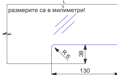
ИЗРЕЗИ НА СЪКЛОТО ЗА ВМ 1049
